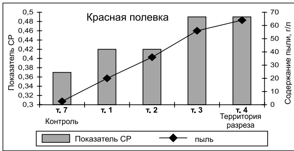
Рис. 1. Нарушение стабильности развития (CP) млекопитающих в окрестностях Кангаласского угольного разреза (т.1–т.7 – точки сбора материала)
