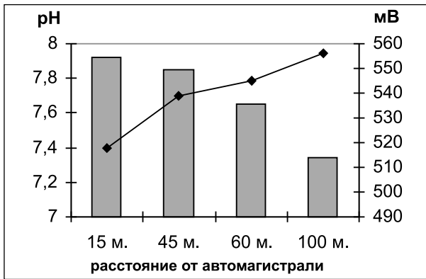
Рис. 2. Значения рН и ОВП почв при удалении от автомагистрали Московская.
