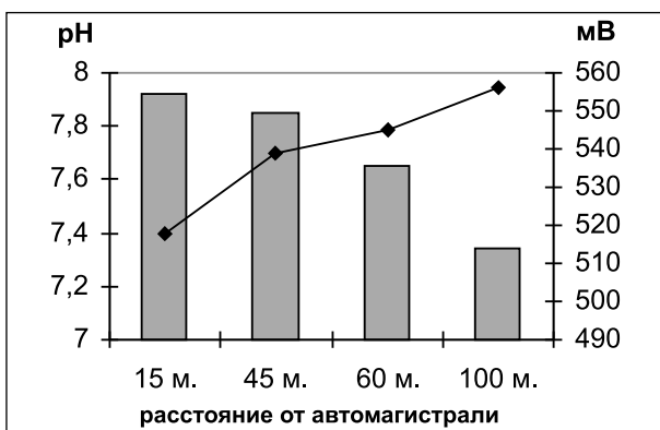
Рис. 2. Значения рН и ОВП почв при удалении от автомагистрали Московская.
